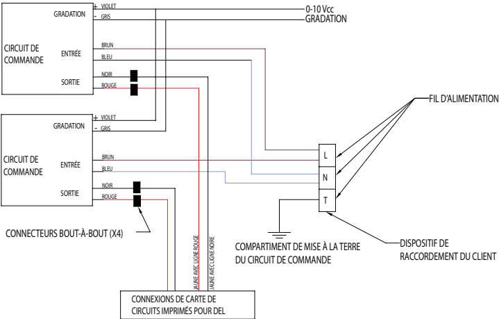
SCHÉMA DE CÂBLAGE CONFIGURATION DE 11L CONFIGURATION DU CIRCUIT REDONDANT S892 DE 5L/7L/9L
