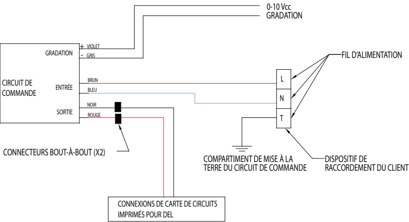
SCHÉMA DE CÂBLAGE CONFIGURATION DU CIRCUIT DE COMMANDE DE 3L/5L/7L/9L
