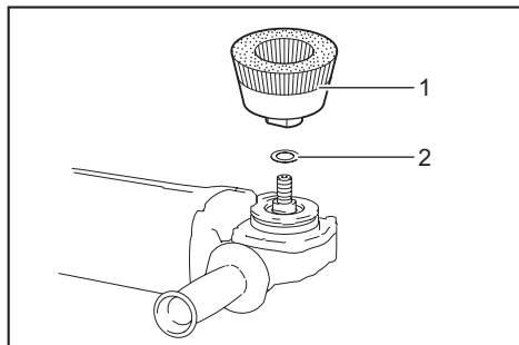
► 1. Brosse coupe métallique 2. Rondelle d'urétrane (comprise dans certains pays)
